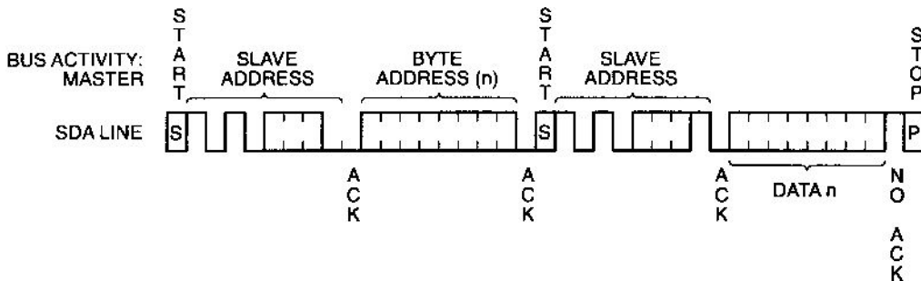
图 10 选择地址读
