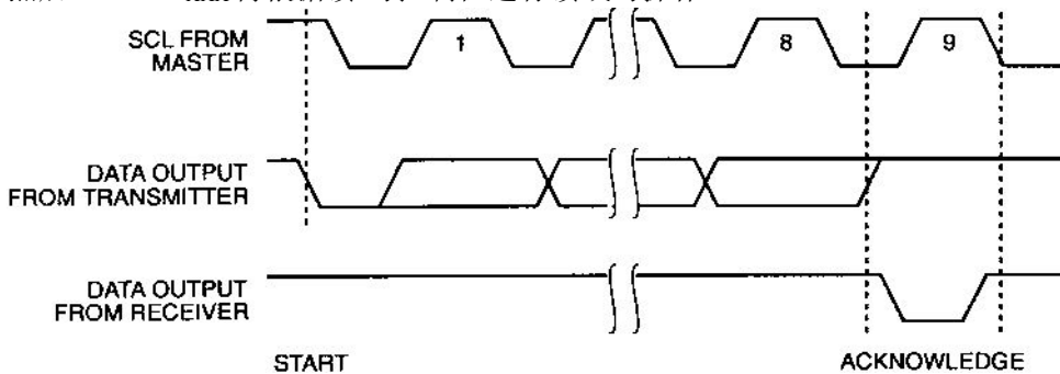
图 5 应答时序
