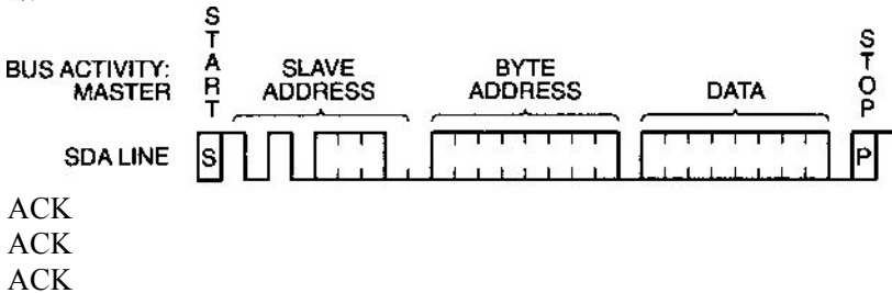
图 7 字节写时序
