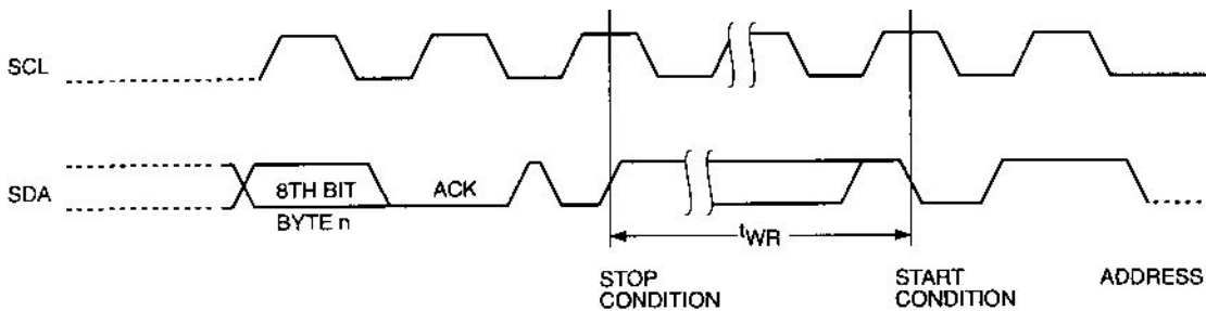
图 3 写周期时序
