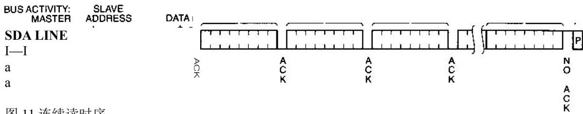
图 11 连续读时序 订单信息
